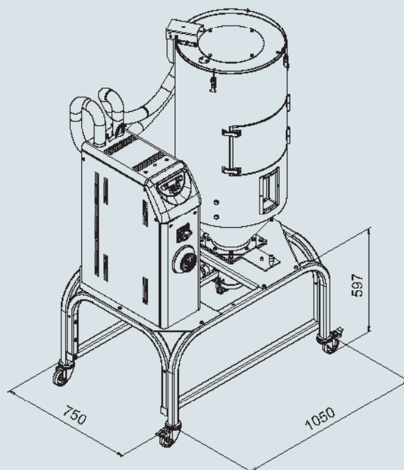
Sistema de deshumidificación monotolva sobre carro T 75 ÷ T 200
