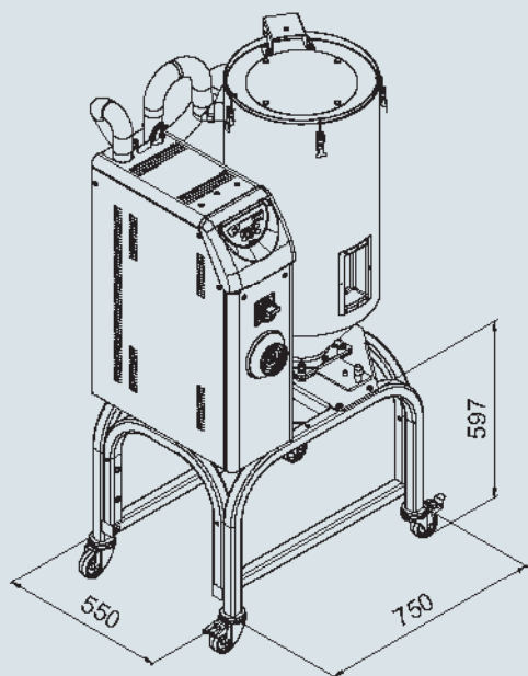
Sistema de deshumidificación monotolva sobre carro T30 ÷ T50
